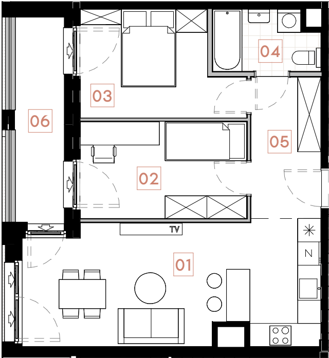
RZUT LOKALU 42
