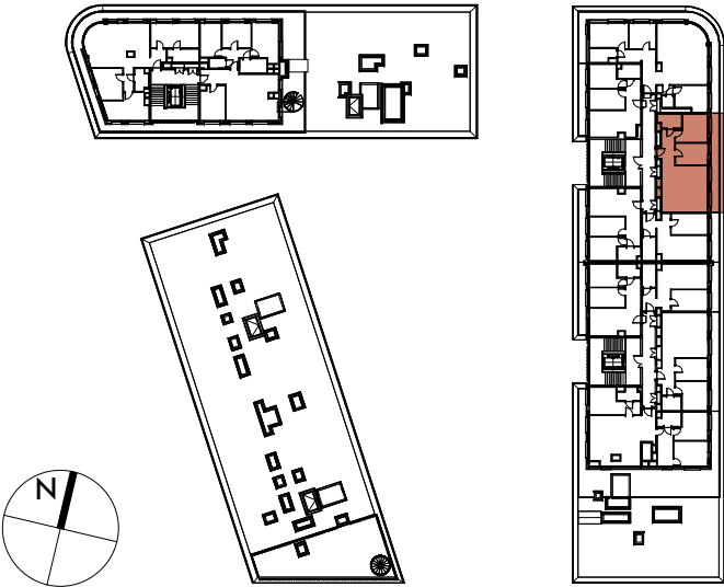
BUDYNEK B1.1 | RZUT KONDYGNACJI 07
