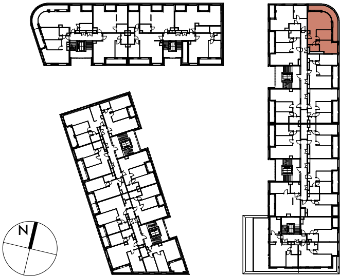
BUDYNEK B1.1 | RZUT KONDYGNACJI 04
