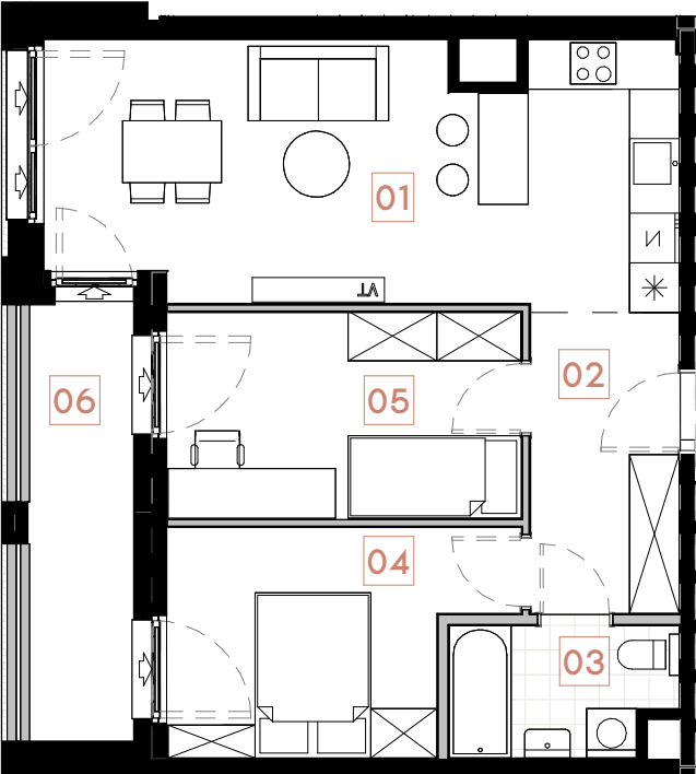
RZUT LOKALU 10
